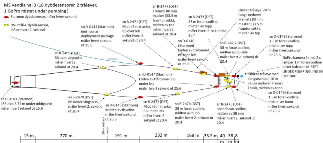
Figur 13. Trålinstrumentering, hal 3
