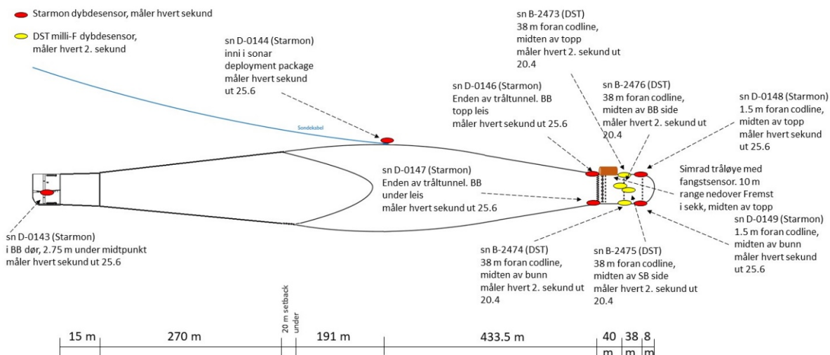
Figur 9. Trålinstrumentering, hal 1
