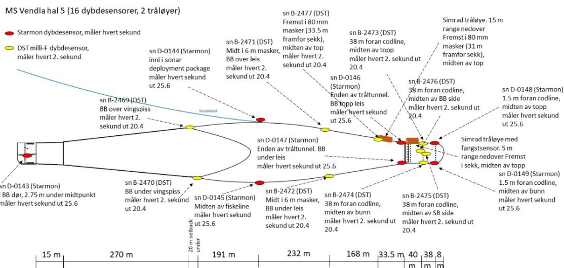
Figur 20. Trålinstrumentering, hal 5
